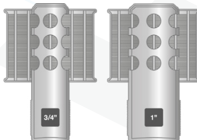
Interior de una tobera tipo Johnson E-I
